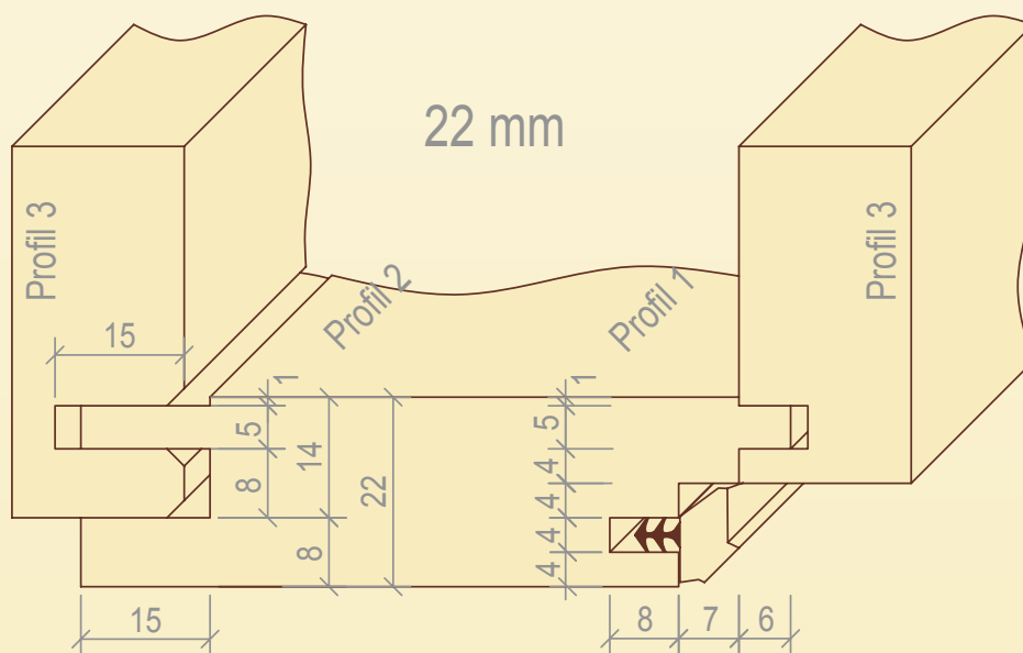
Řez obložkové zárubně
